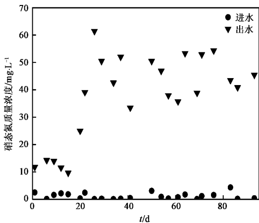
图4 蚯蚓生态滤池进出水NO 3 - -N和NO 2 - -N浓度变化
