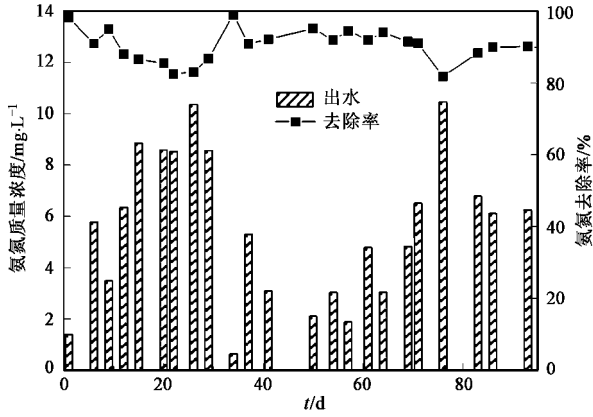
图3 蚯蚓生态滤池对NH 4 + -N的去除效果
